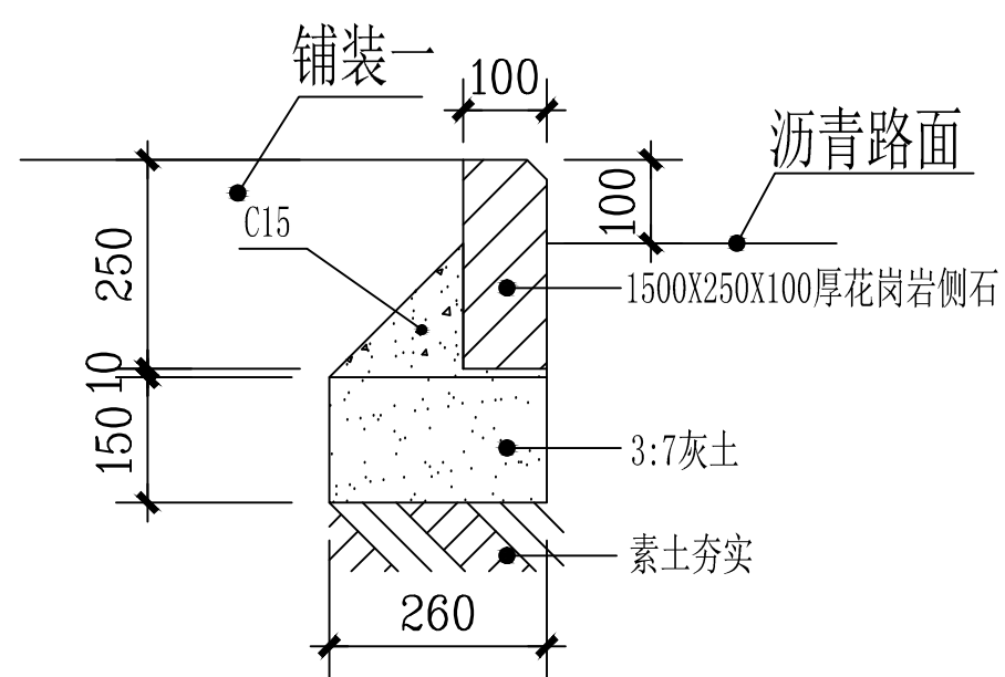
花岗岩侧石做法 1:20
