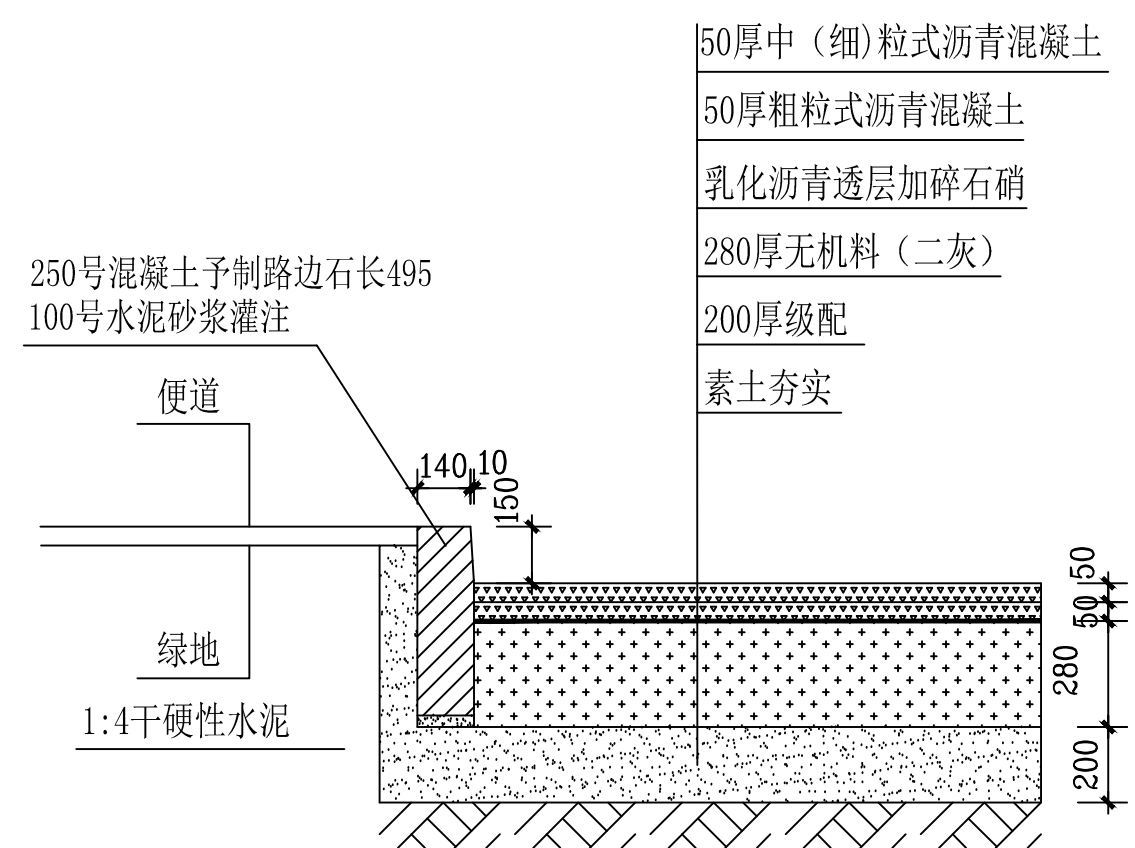
沥青路面做法 1:20
