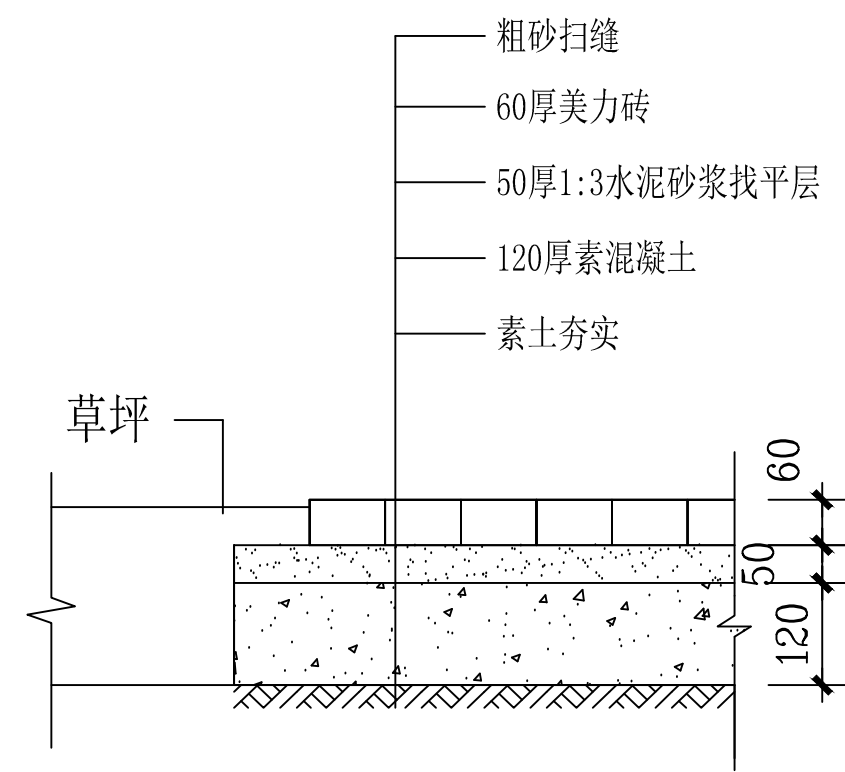
便道做法 1:20
